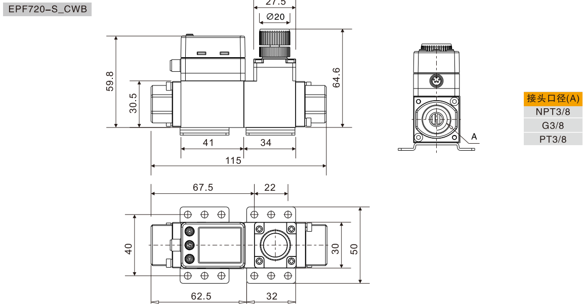
外形尺寸图 (mm)
