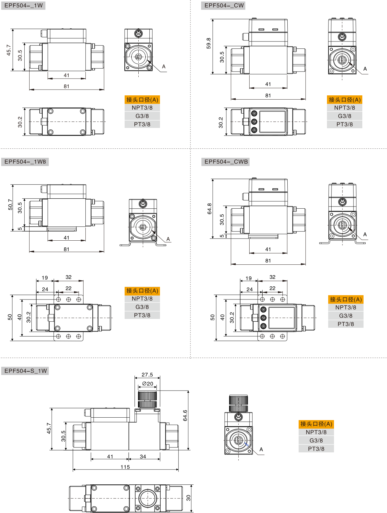
外形尺寸图 (mm)
