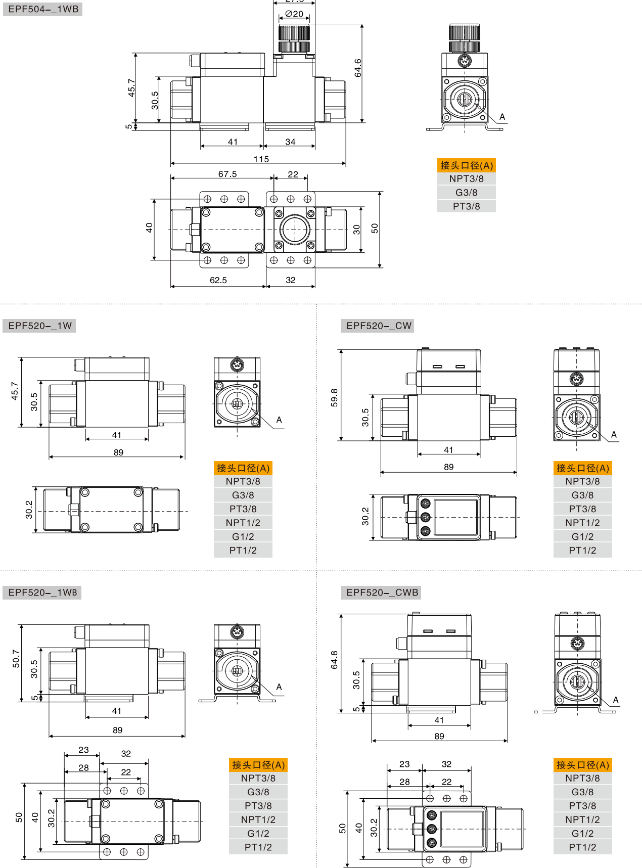
外形尺寸图 (mm)
