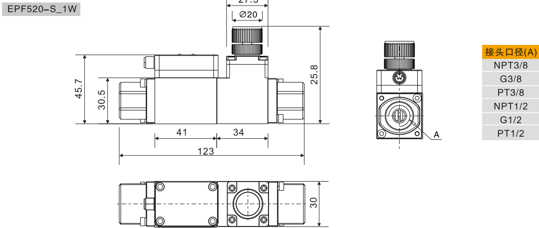
外形尺寸图 (mm)
