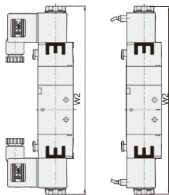
接线盒式
