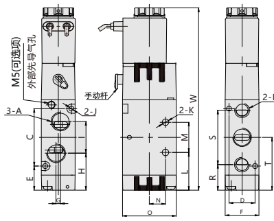
引出线式
