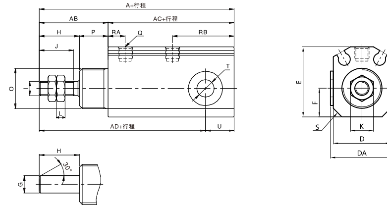
无牙活塞杆
