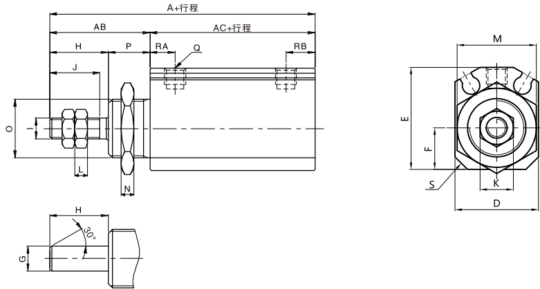
无牙活塞杆
