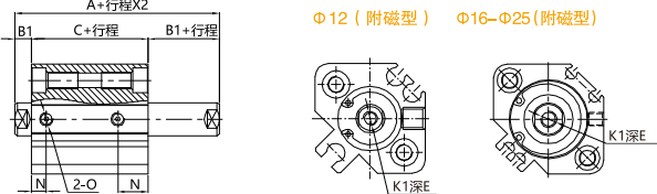
SQNDØ12~Ø25 (附磁型)
