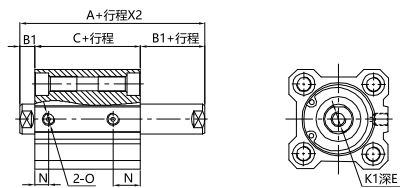
SQNDØ12~Ø25 (不附磁型)
